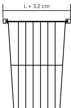
Korgens höjd 48 cm
